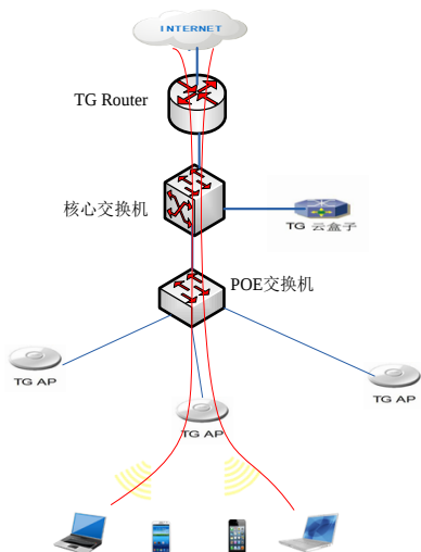
图 3-1-18 AP 本地转发模式数据流
